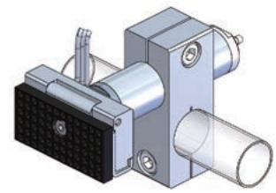
Gripper module • for jungle gym ( \phi 20)
