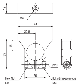
Tie wrap base \phi 20 (M4)
