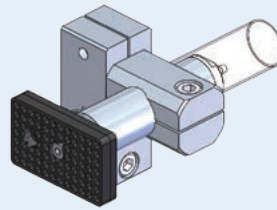
Gripper module • for jungle gym (φ 20)
