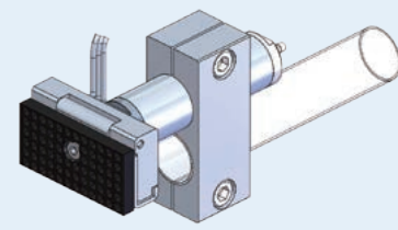
Gripper module • for jungle gym (φ 20)
