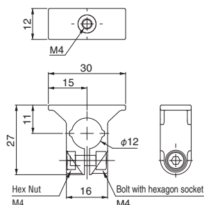
Tie wrap base \phi 12 (M4)
